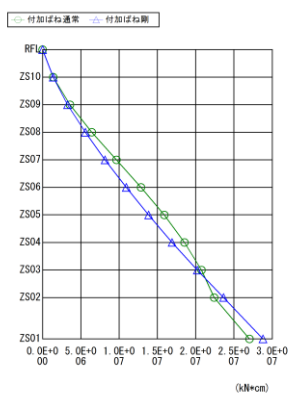
重心の最大応答回転モーメント
