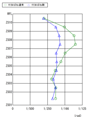
重心の最大応答層間変形角
