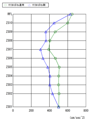
重心の最大応答絶対加速度
